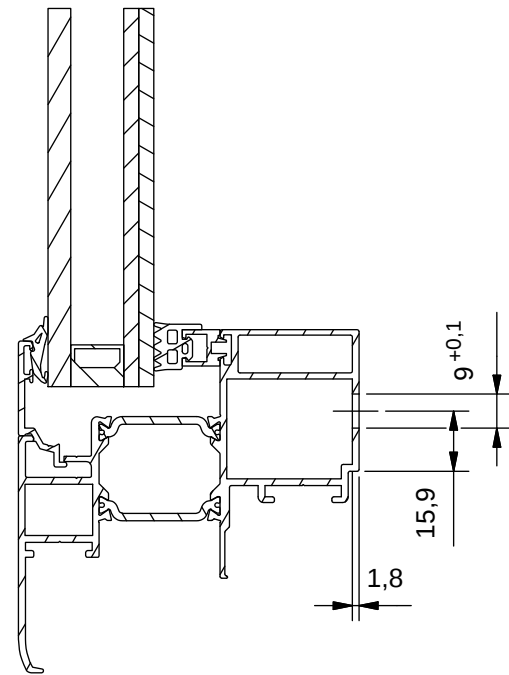
Flügelrahmen / sash-frame: 0071768
