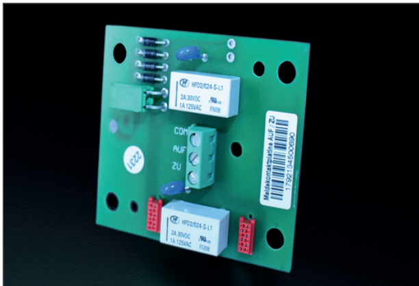
Meldekontakt AUF/ZU
