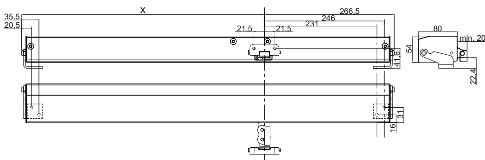
WMU 86x/88x-n + WAB 836B 01 + WAB 836E 01
