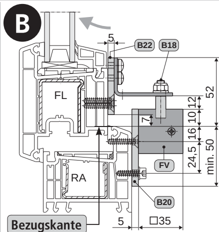
Darstellung am Kunststoff-Fenster
