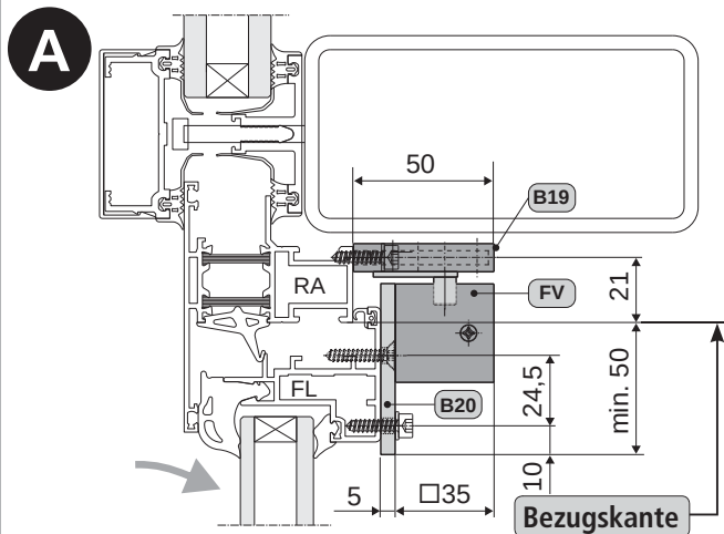
Darstellung am Alu-Fenster
