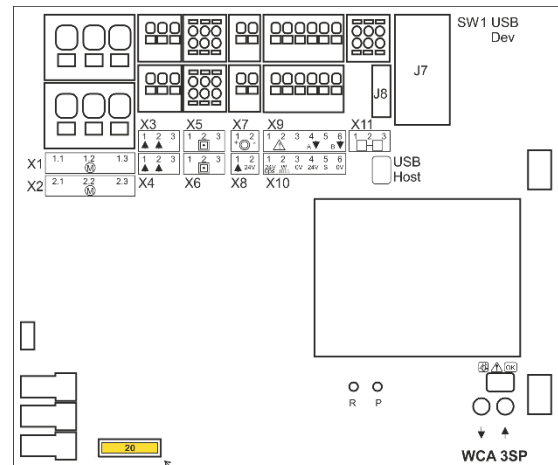
20A Flinke Sicherung Platzierung der 20A (flink) Sicherung
