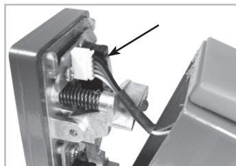
Den Gehäusedeckel langsam öffnen und dabei das Kabel des Funksenders abziehen.
