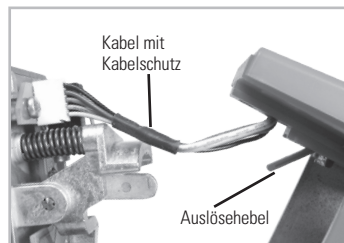
Wenn der Gehäusedeckel geschlossen wird, muss der Auslösehebel komplett ausgeklappt sein und das Kabel seitlich liegen.
