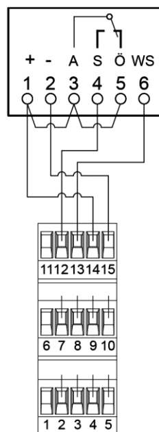
Modulo di ventilazione MZ3
