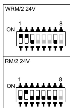
DIP-Schalteneinstellung
