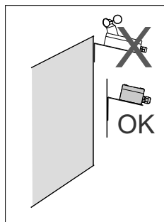
Nástěnná montáž
