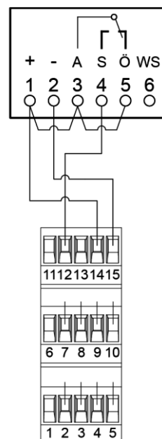
MZ3 Lüftungsmodul LM
