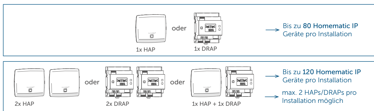
Abbildung 1: Kombination und Limits von Access Points
