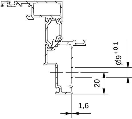
Flügelrahmen / sash-frame: 270 209
