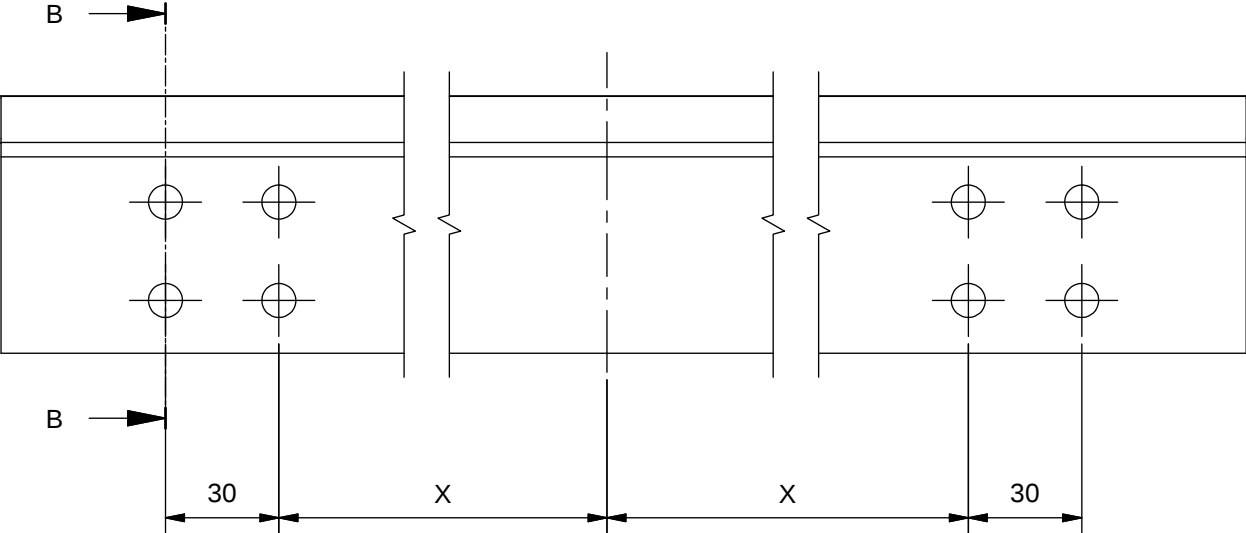
Bohrbild 2 passend für Einspannrahmen 270125 / Drilling template 2 fits for insert unit 270125 für Rahmenkonsole / for Frame bracket: CDP-FB002
