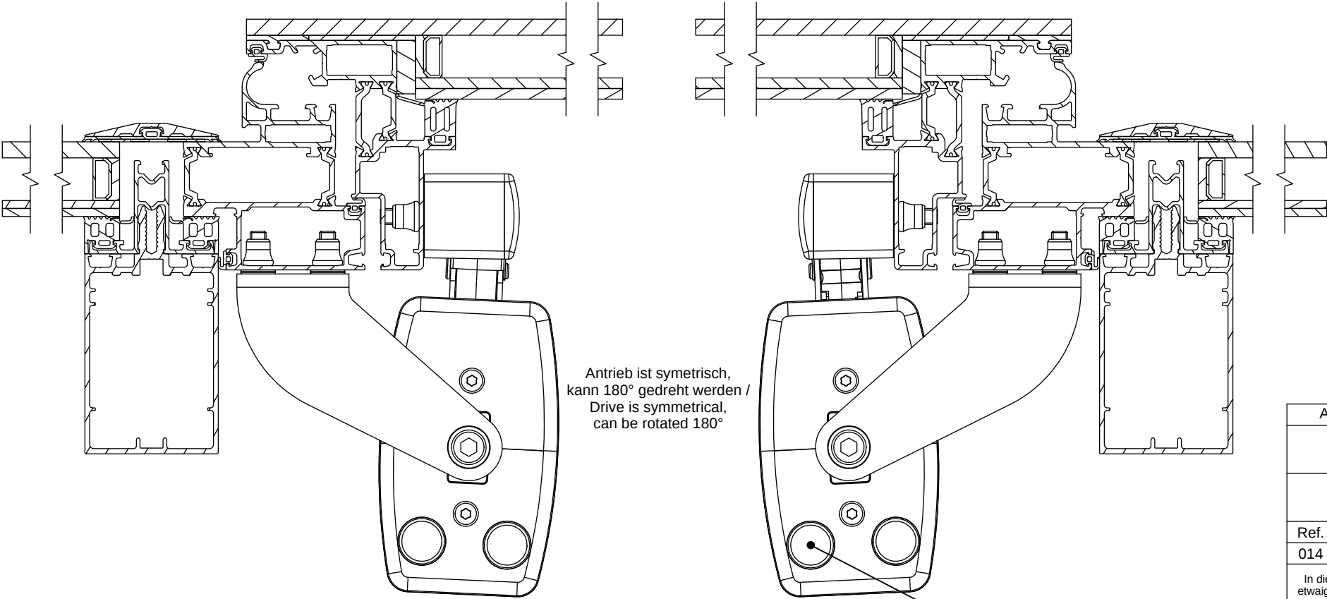
A-A ( 1 : 2 )
