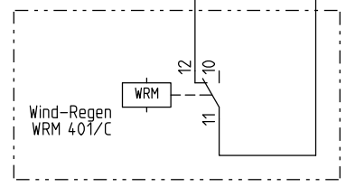
Anschluss (W)RM 401/C (nur potentialfreie Kontakte)
