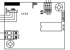
Wind-/ Regen- Fühler WRF 501
