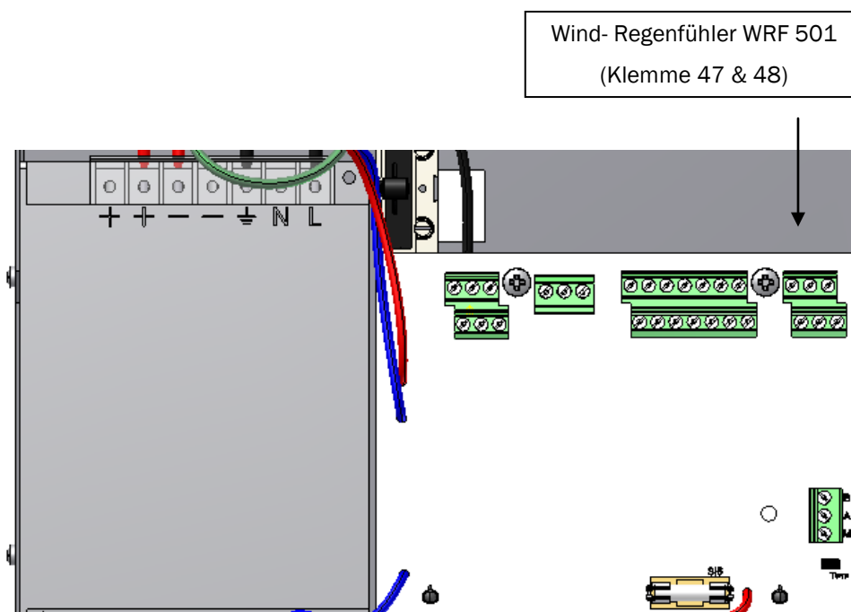
Abbildung 6: Anschluss Wind-/ Regenfühler WRF 501 oder Regensensor RS 501
