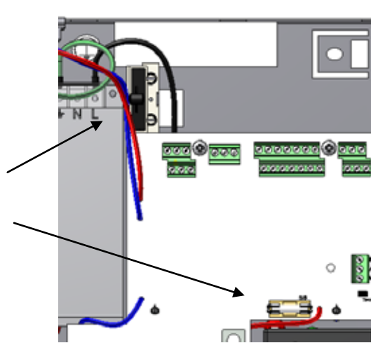
Abbildung 12: Sicherung auf der Platine
