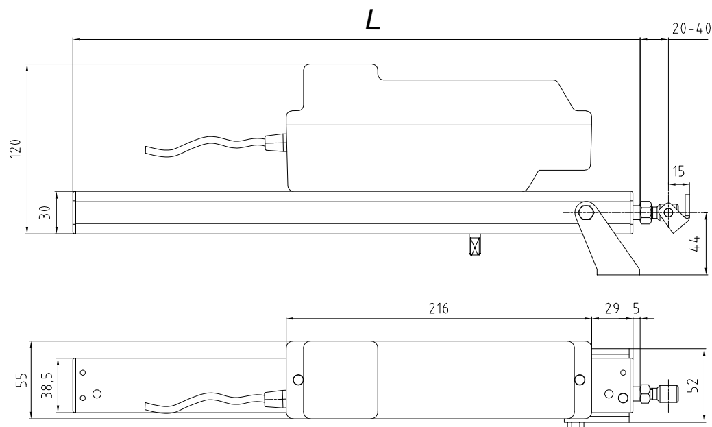
ATTUATORE CON STAFFA SCORREVOLE COD. 40235F ACTUATOR WITH SLIDING BRACKET COD. 40235F
