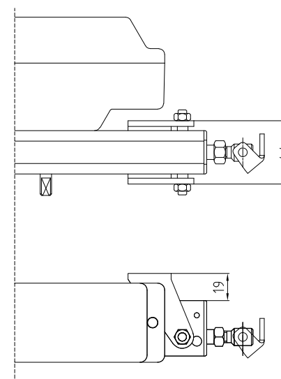
ATTUATORE CON STAFFA FISSA COD. 40234E ACTUATOR WITH END BRACKET COD. 40234E
